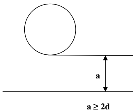
Rysunek 5: Wzajemne usytuowanie otworu i obrzeża szyby
