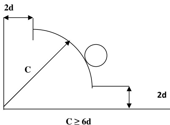
Rysunek 7: Wzajemne usytuowanie otworu i naroża szyby
